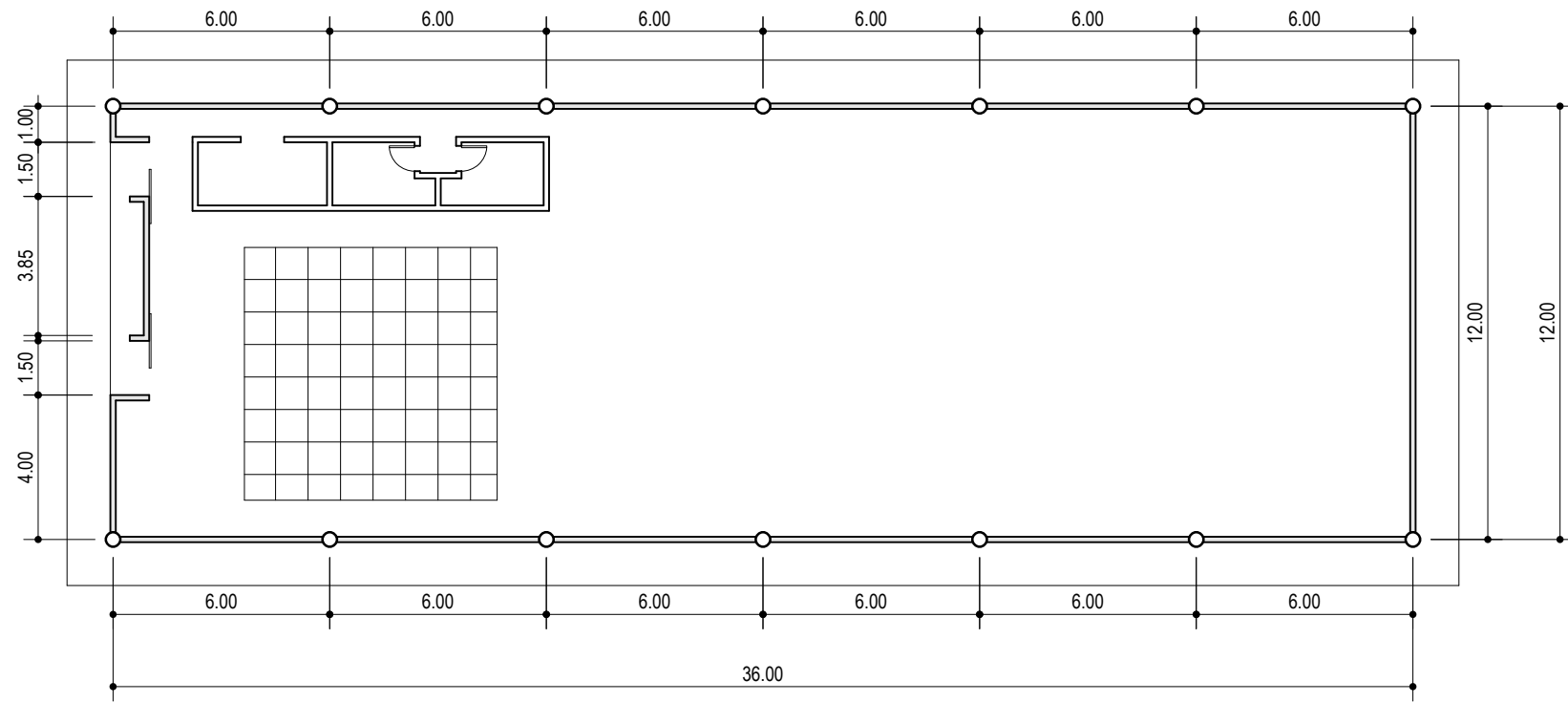
GAU013: PLANTA DE GALPÃO ESCALA: 1:200 [Dim. metros]
